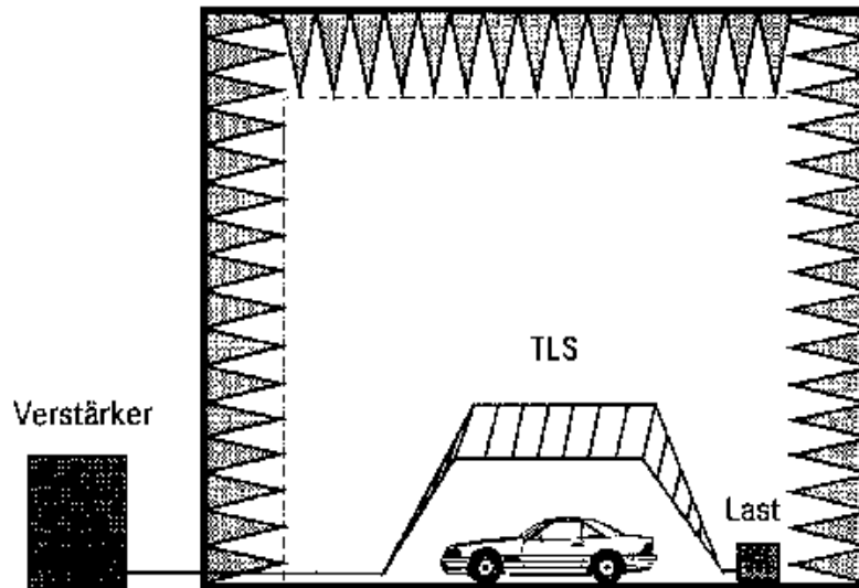
Prüfaufbau: Einstrahlung mit einem TLS
